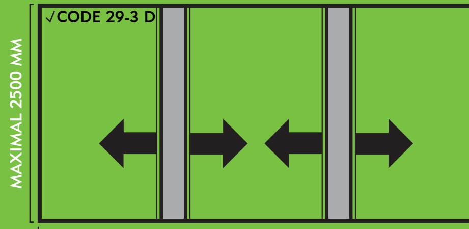
MAXIMAL 3001 MM – 4000 MM DOPPELTES REVERSIBLES PLISSEE
