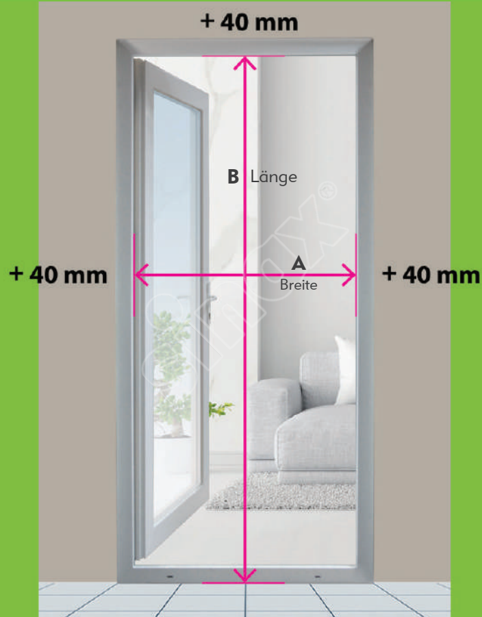
Drehtürsystem
